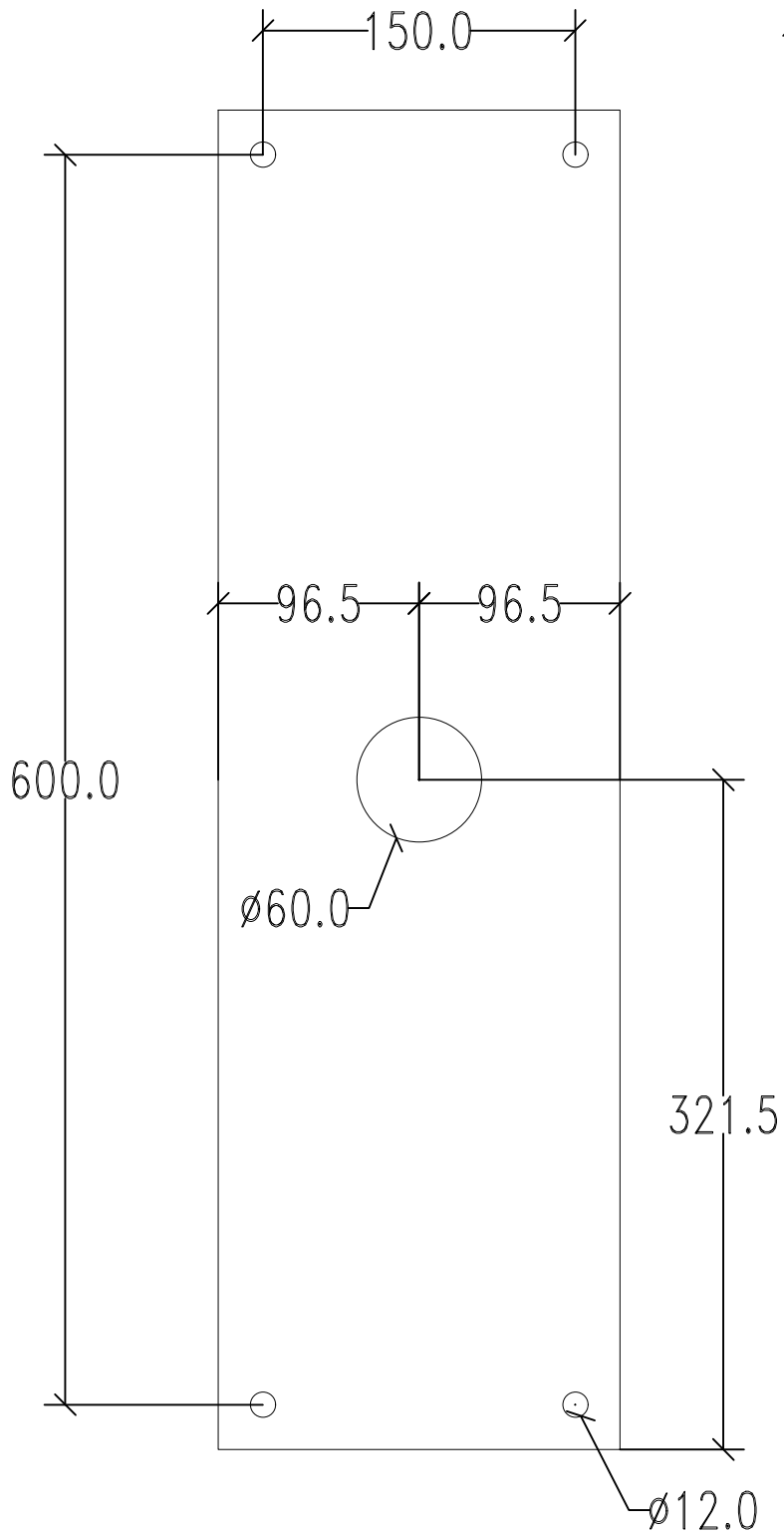
hole templates
