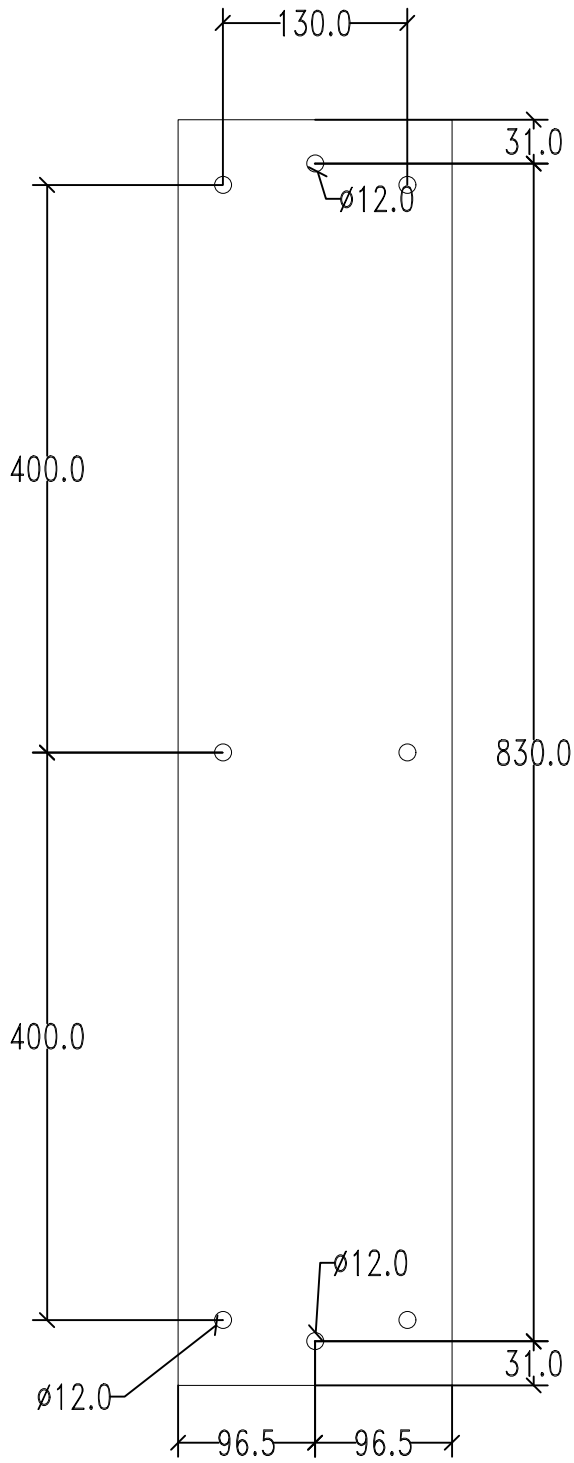
hole templates
