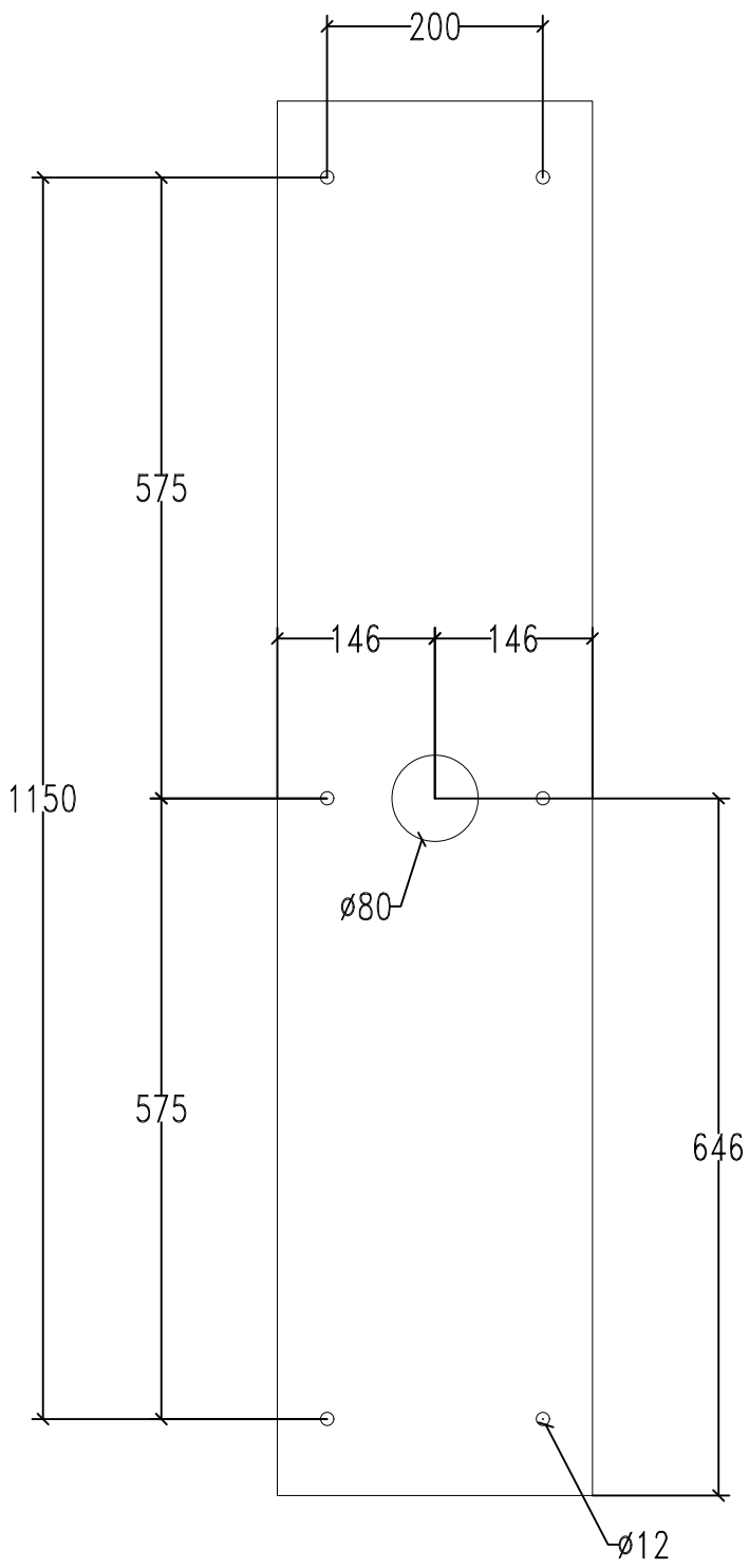
hole templates
