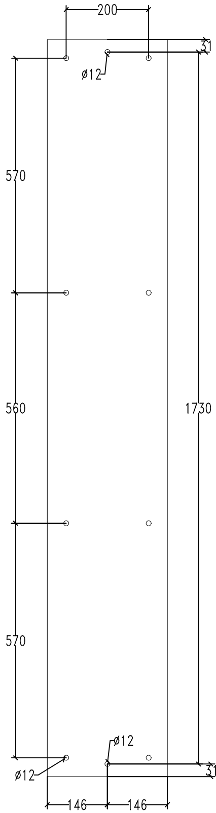
hole templates
